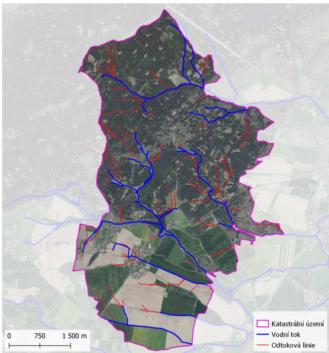
Obr. 10: Odtokové linie s plochou sběrného povodí > 5 ha na území obce Rosovice
