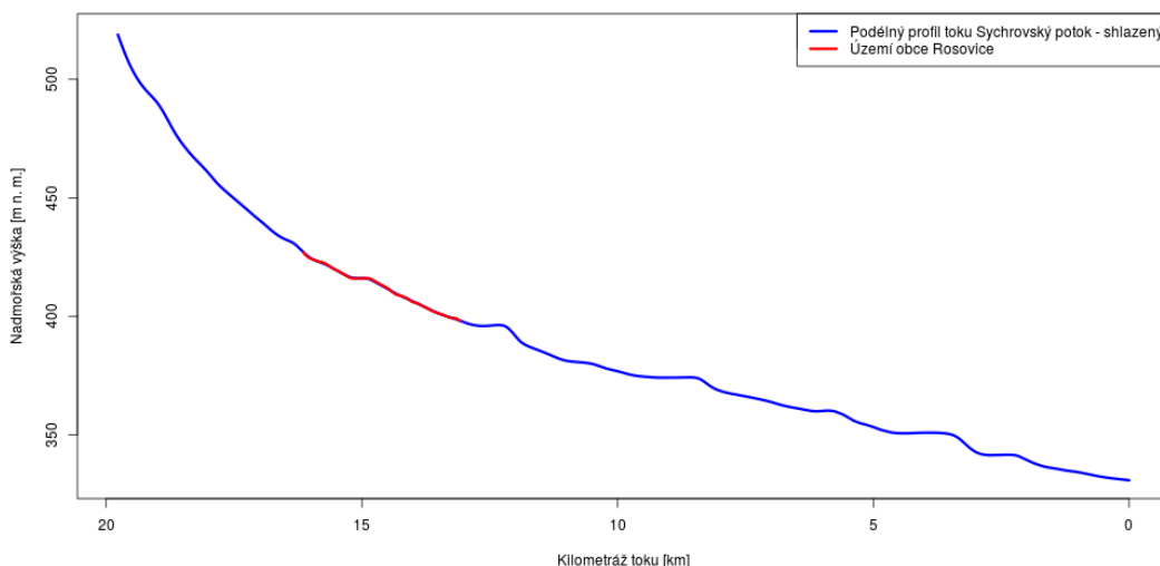
Obr. 5: Podélný sklon vodního toku Sychrovský potok
